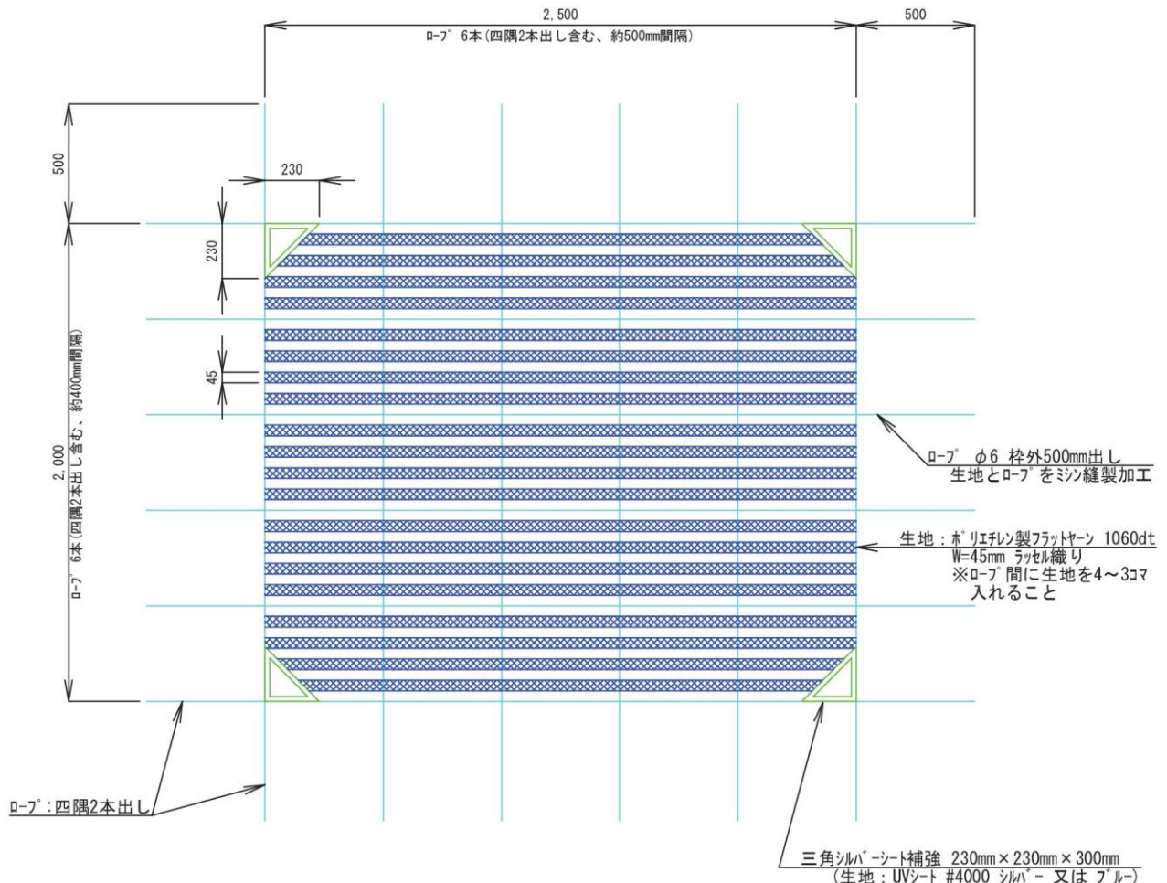
【指定品】吹溜り防止柵用ネット寸法図 (S=FREE)
