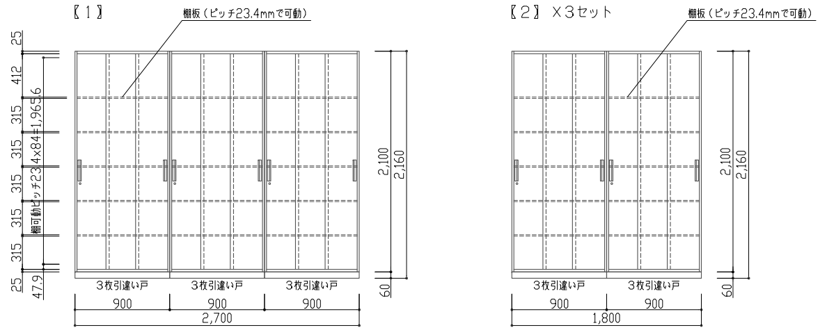
■ 収納庫展開図
