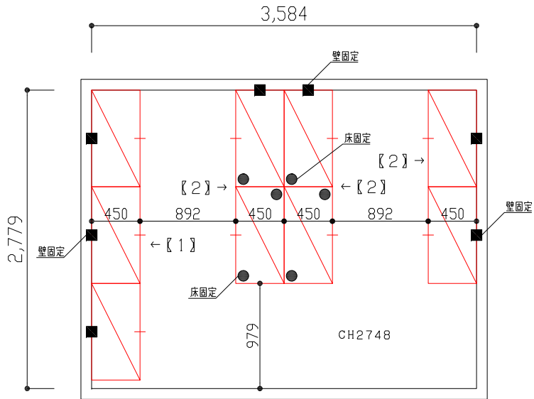
■ 収納庫配置図（収納庫台数：9台）
