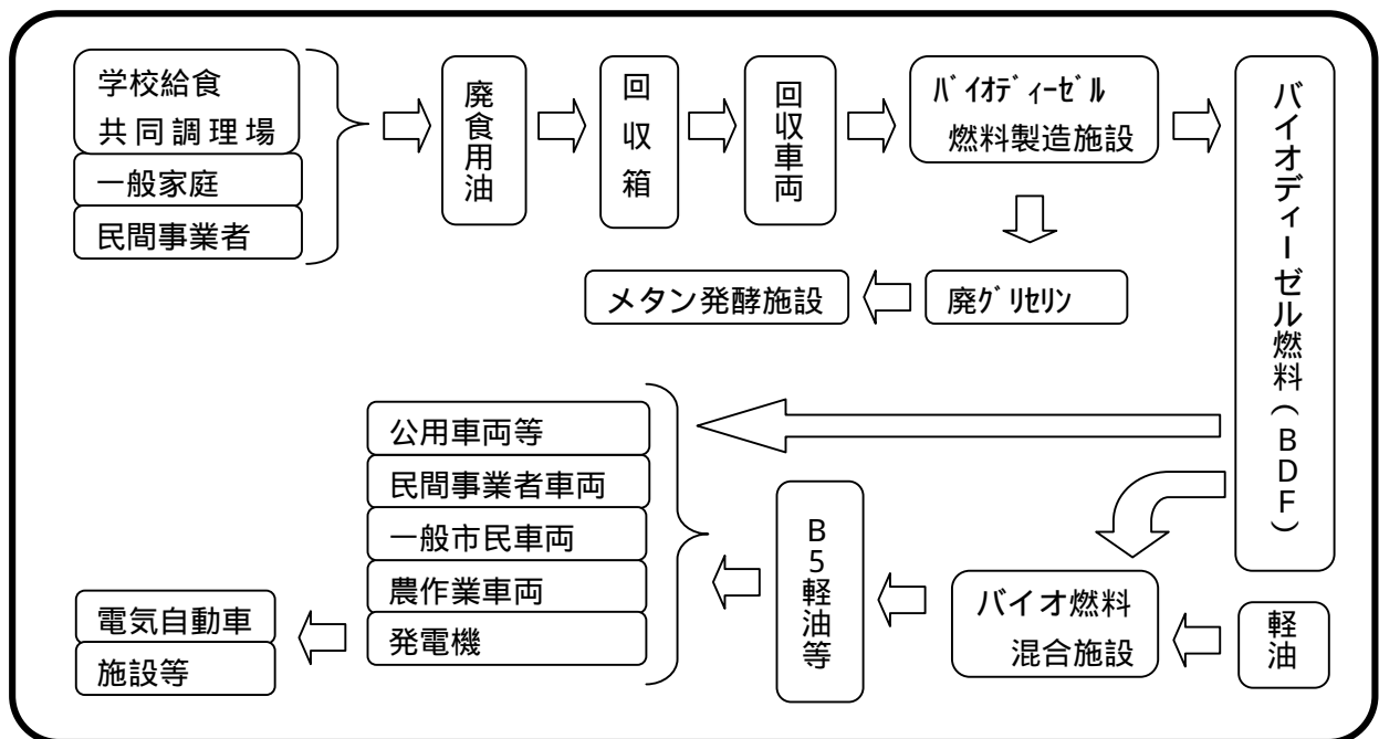
図 6 . バイオディーゼル燃料事業のイメージ図
