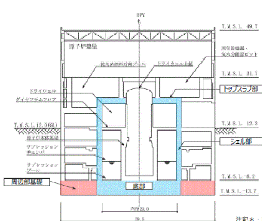
原子炉建屋の断面図
