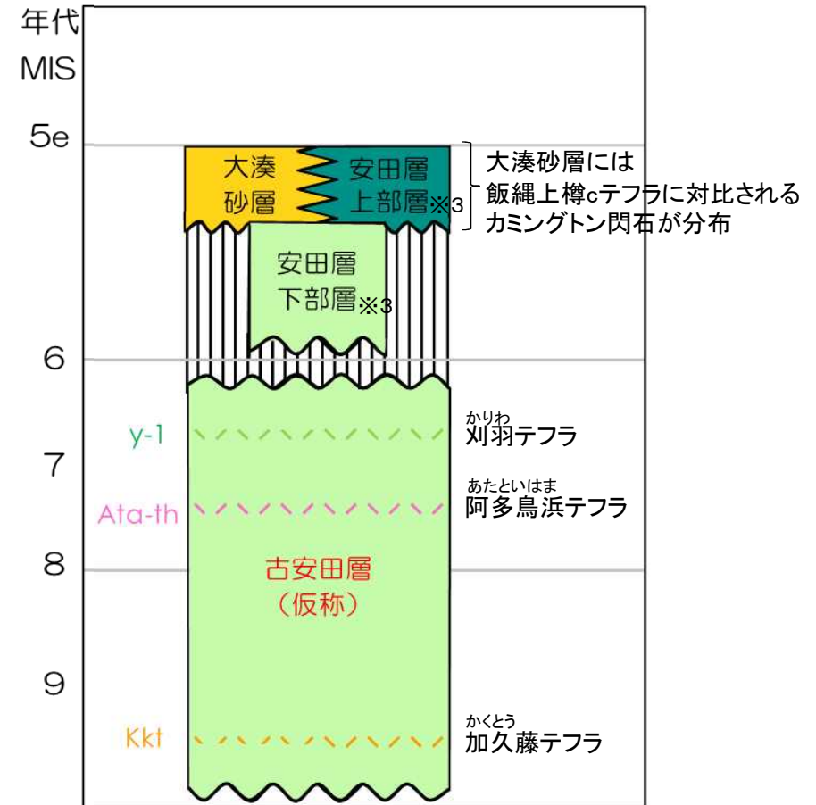
【模式柱状図】
