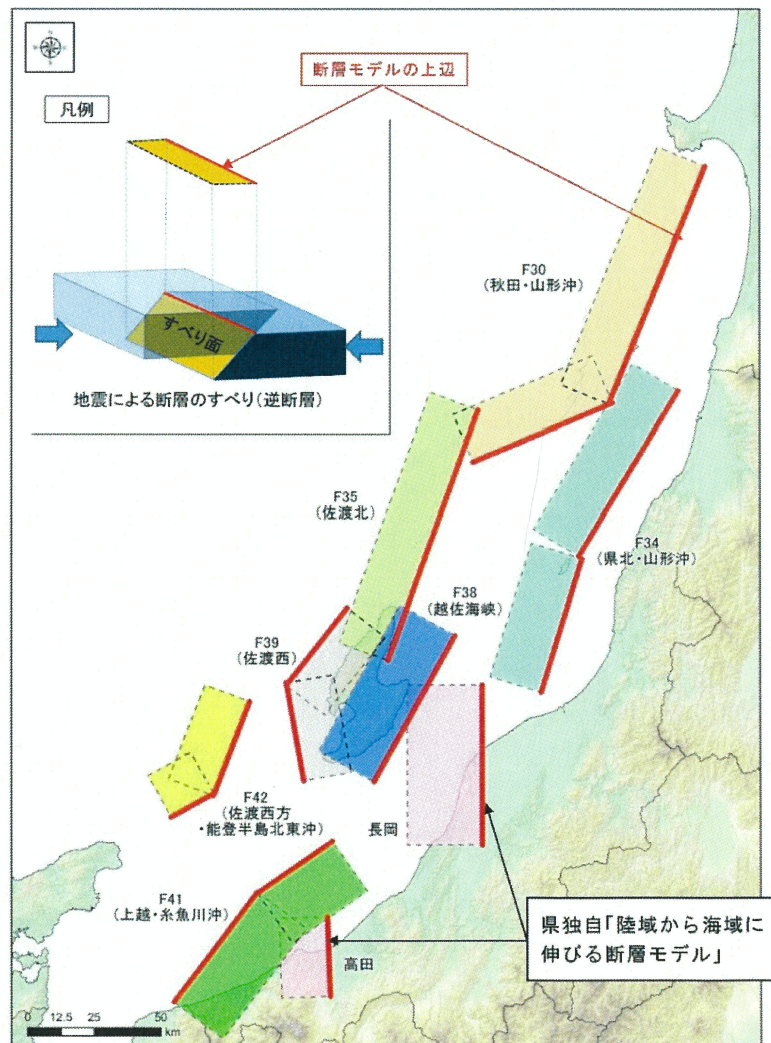
図 1.1 津波断層モデル位置図
