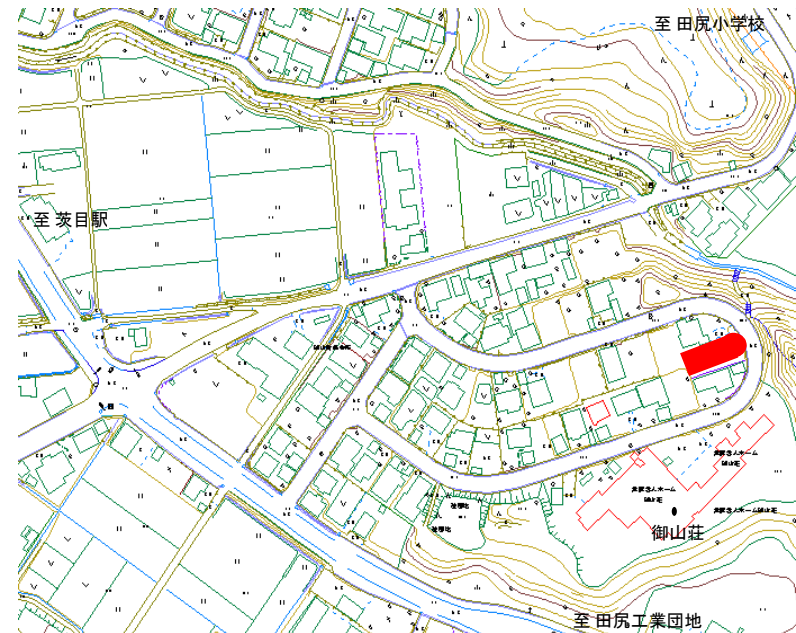
明細図
